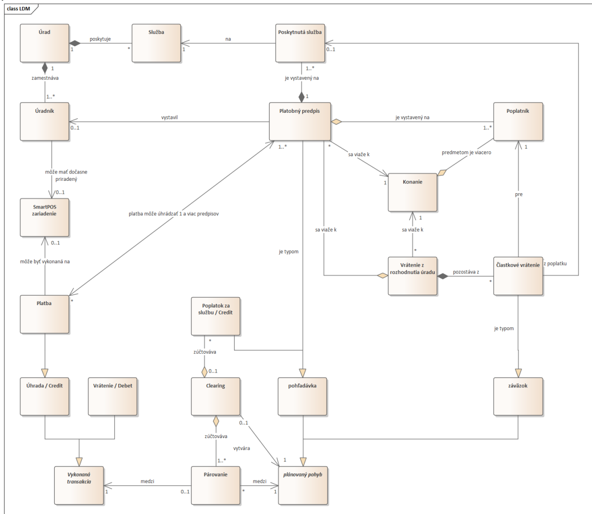
Obrázok 8: Logický dátový model nového riešenia
