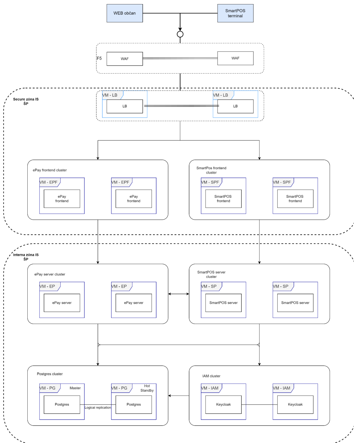
Obrázok 9: Technická architektúra
