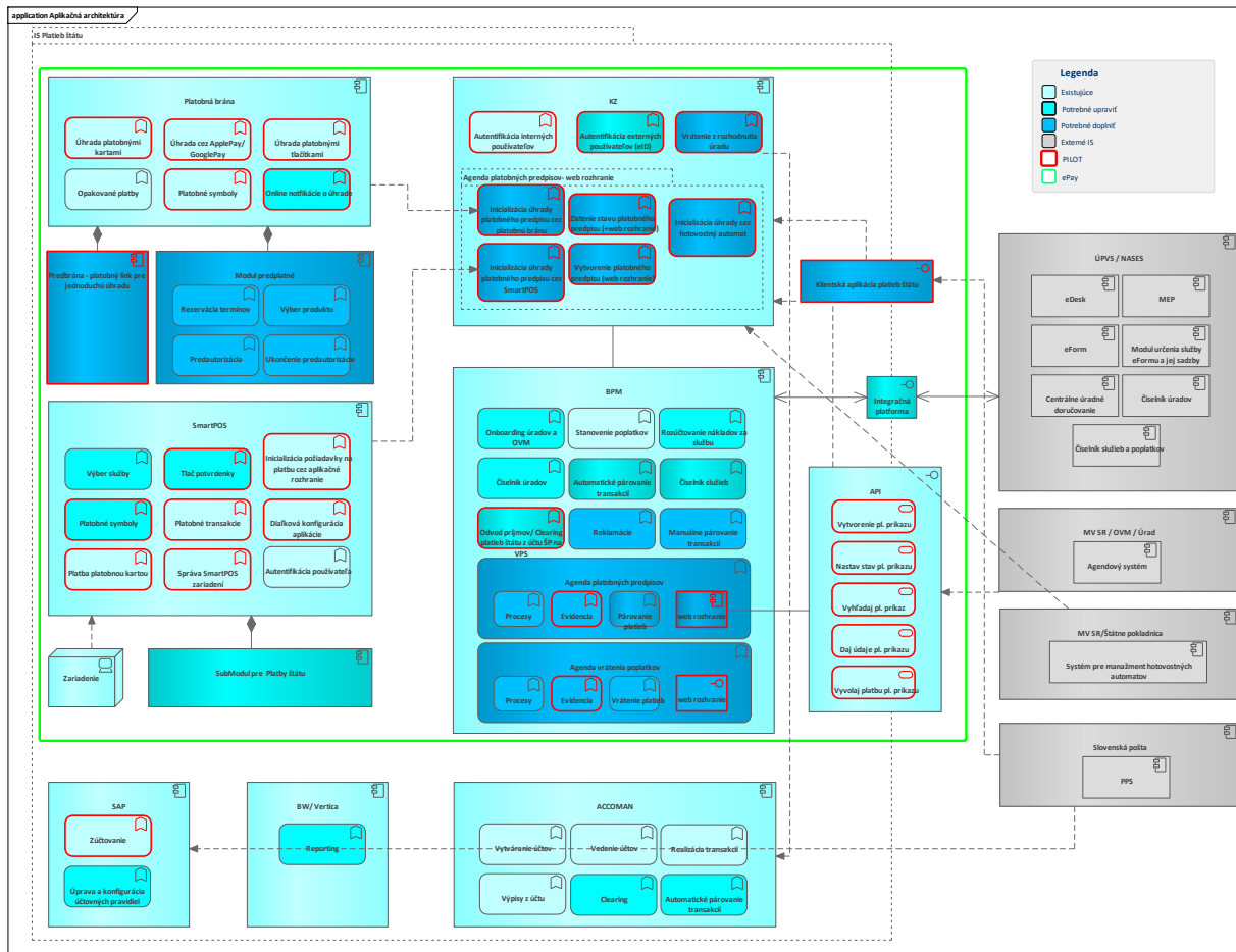
Obrazok 7: Aplikačná architektúra nového riešenia
